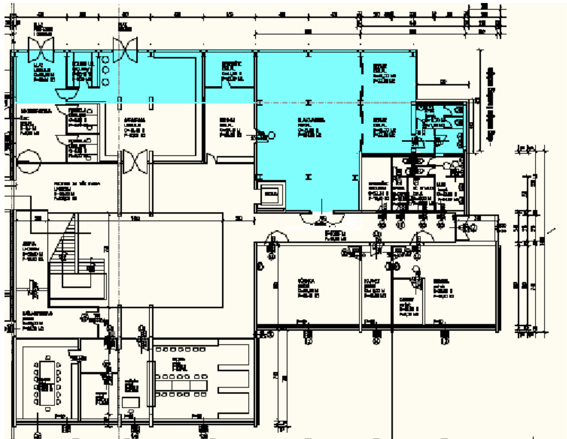
TLOCRT PRIZEMLJA - ISTOK
