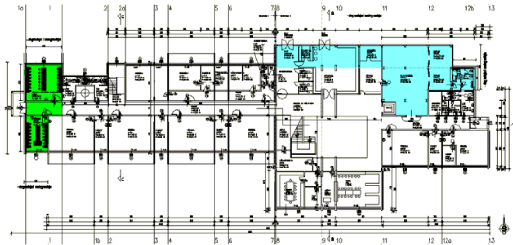
TLOCRT PRIZEMLJA MJ 1:200
